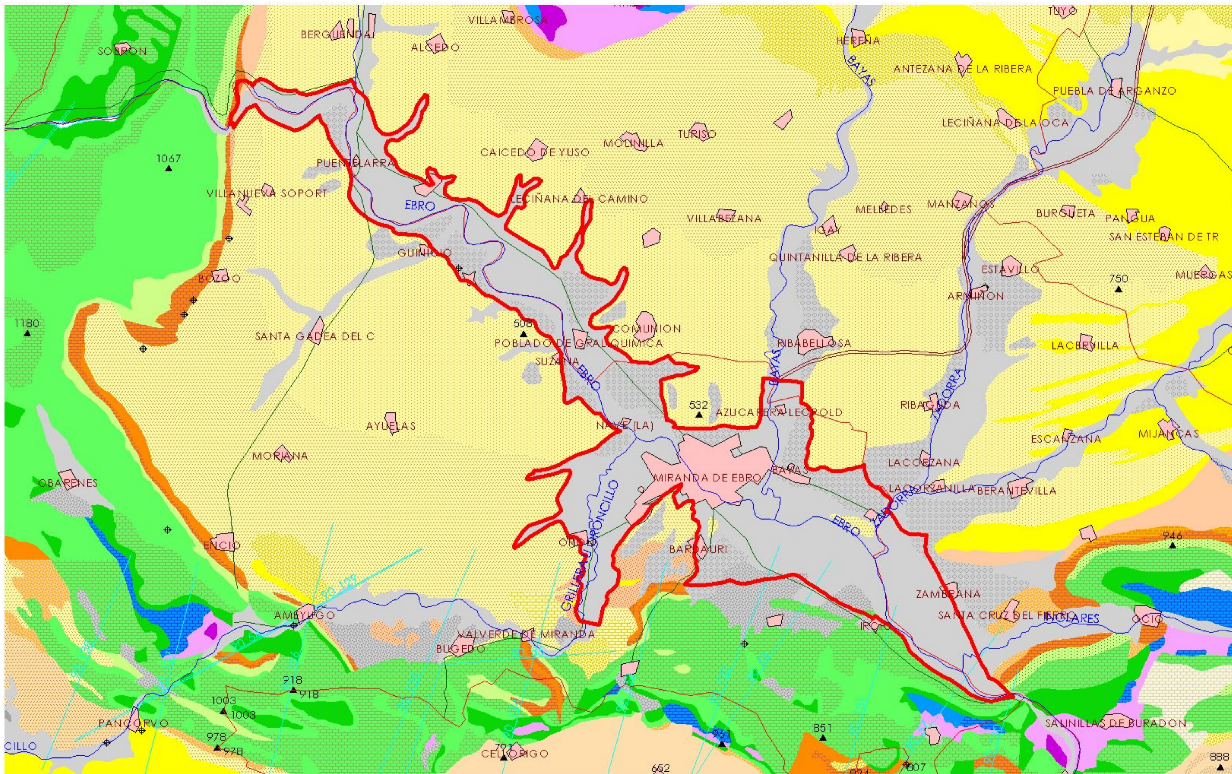
MAPA 2.1; MAPA GEOLÓGICO 90_009 ALUVIAL DE MIRANDA DE EBRO
