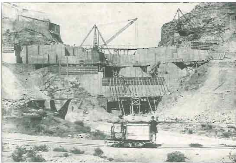
Vista del paramento de aguas arriba, en el estado actual de las obras.
