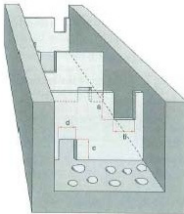
Fig. 12. Vista de una escala de estanques sucesivos. (Larinier 1992)
