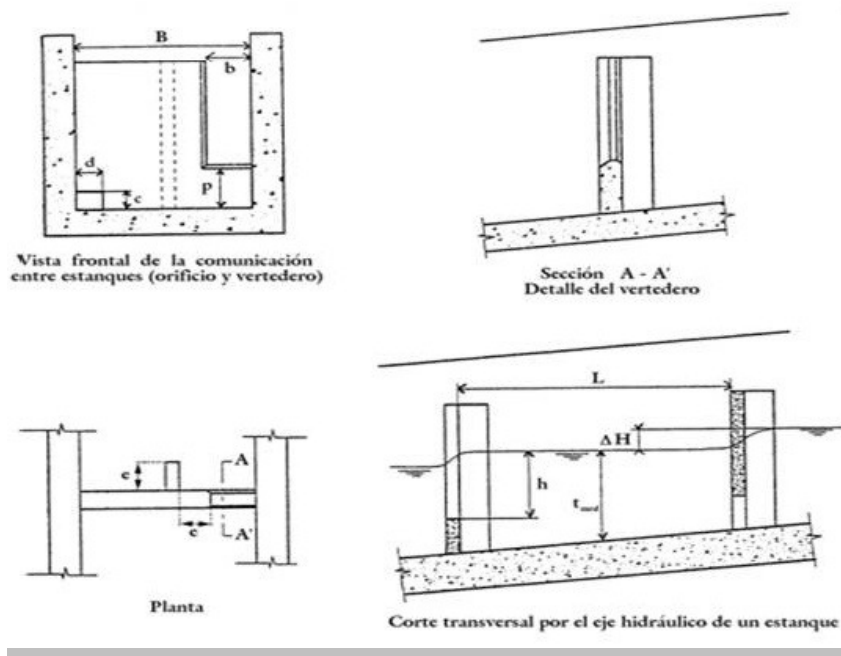
Fig. 13. Esquema de la artesa tipo.
