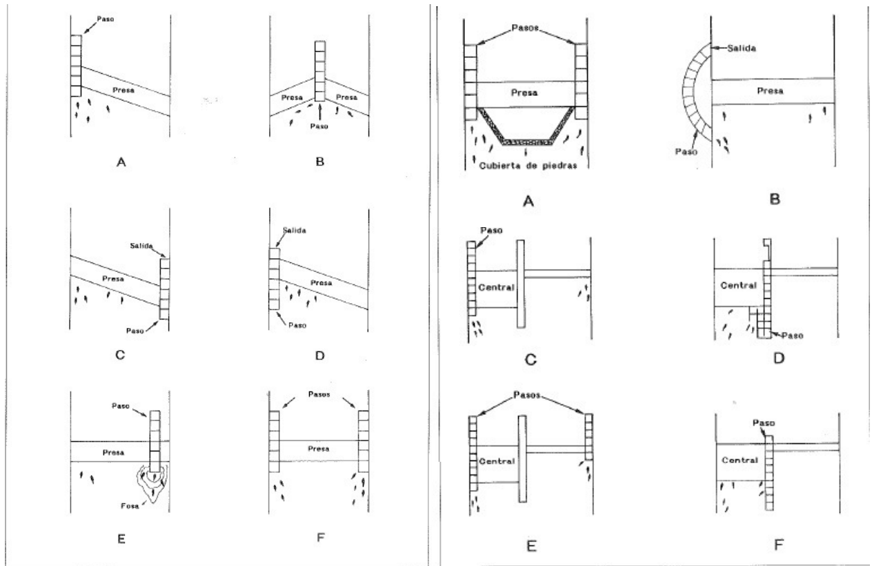
Figura 16. Disposición del paso en el obstáculo. A. Cubierta de piedras bajo el obstáculo para facilitar el acceso de los peces a los pasos. B. Situación del paso cuando existen problemas de espacio junto al obstáculo. C, D y E. Situación correcta del paso en un aprovechamiento hidroeléctrico. F. Situación incorrecta del paso en un aprovechamiento hidroeléctrico.
